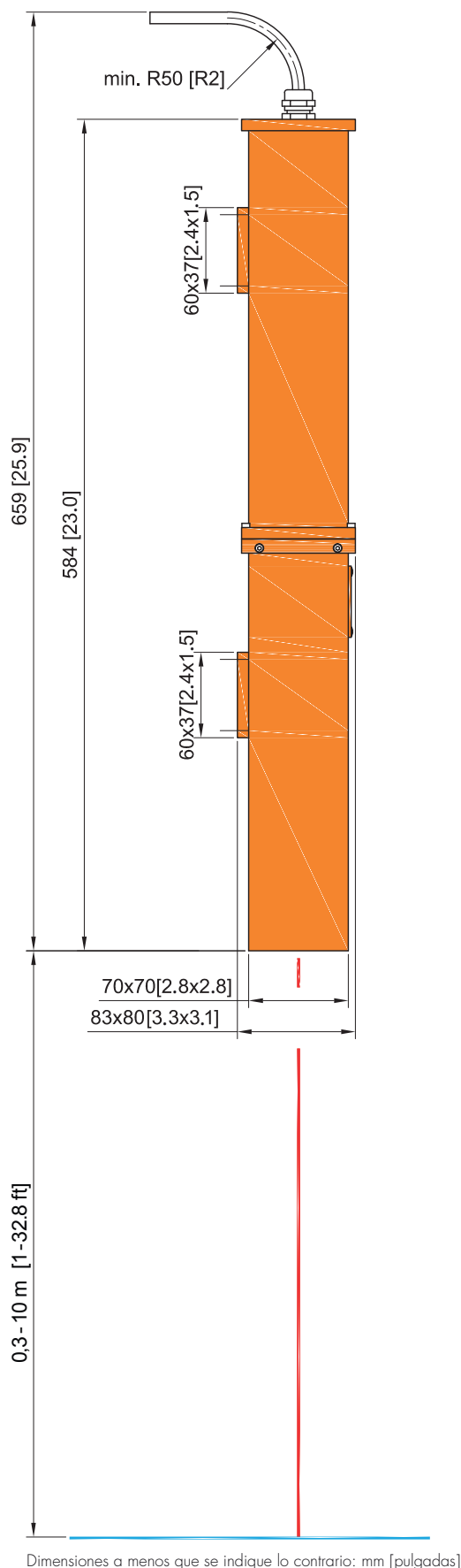
Dimensiones a menos que se indique lo contrario: mm [pulgadas]
